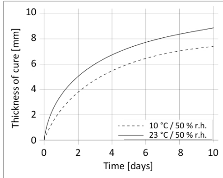
Grafico 1: Velocità di polimerizzazione per Sikaflex®-292i
